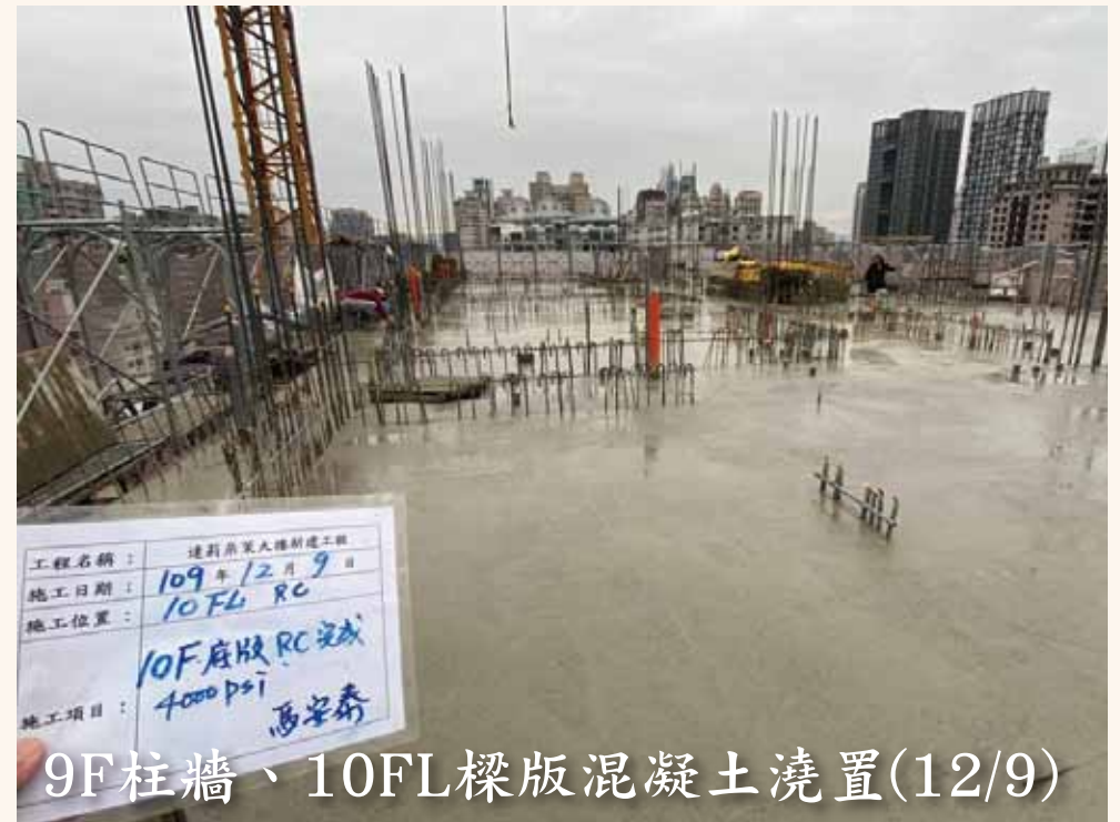
9F柱牆、10FL樑版混凝土澆置(12/9)
